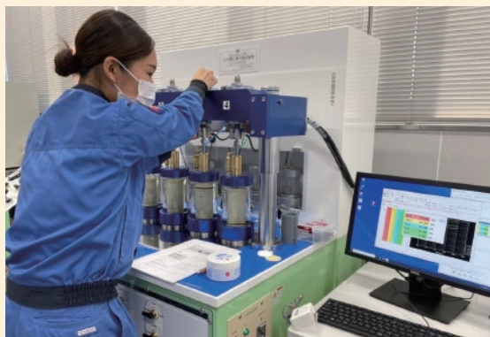
土のCBR試験
