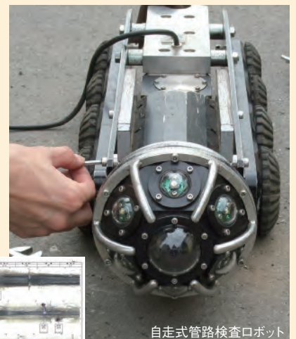
自走式管路検査ロボット
